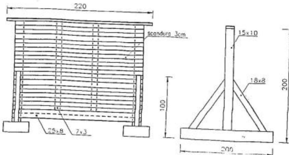
GARDUL DE 2,00m
