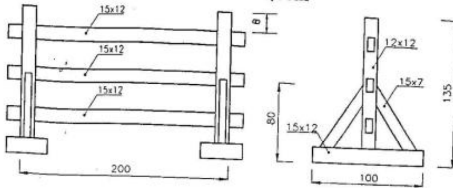
GARDUL DE 1,35m
